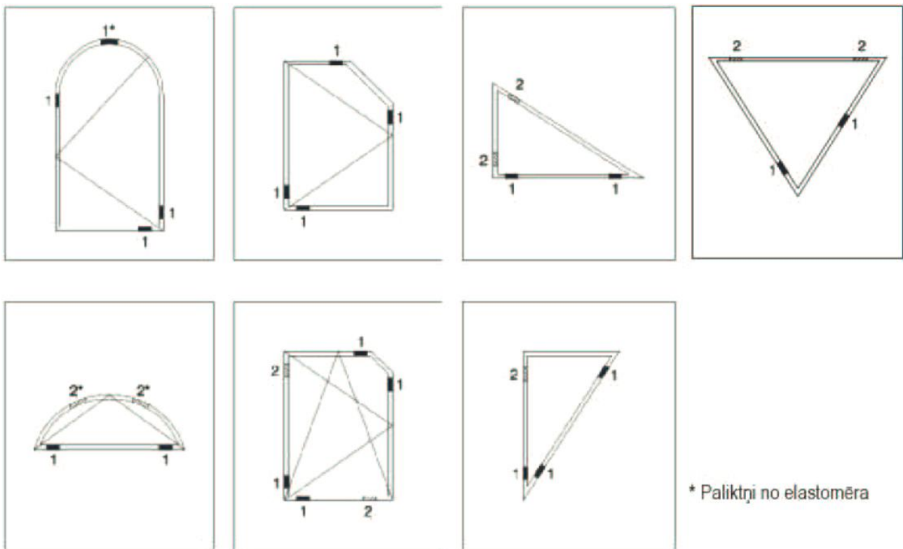
11.zīm. Stiklošanas paliktņu izvietouma shēmas īpašām formām
