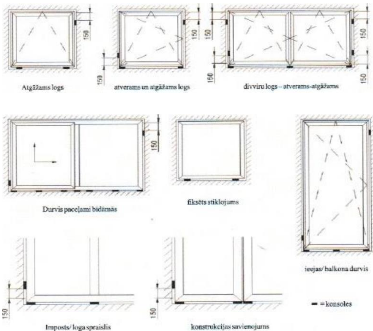
4.zīm. Logu/durvju elementu atbalsta paliktņu izvietojuma shēmu piemēri.
